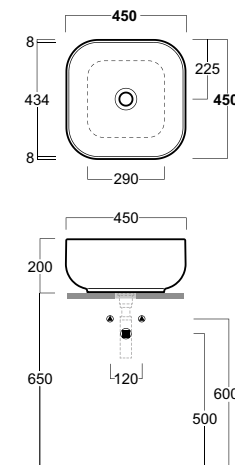
BA 03 Lavabo quadrato d'appoggio Square countertop washbasin 45.45.h20
