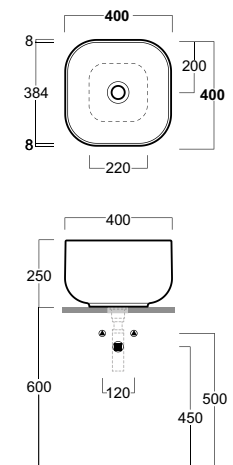
BA 04 Lavabo quadrato alto d'appoggio Square countertop washbasin with high rim 40.40.h25
